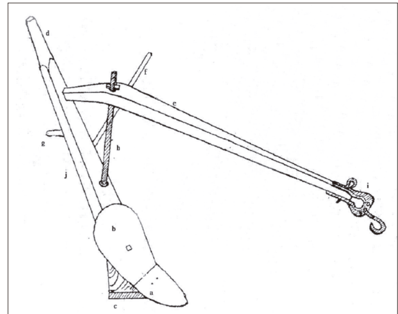
圖三、改良犁
