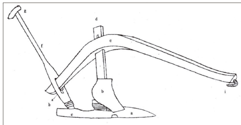
圖二、臺灣在來犁
