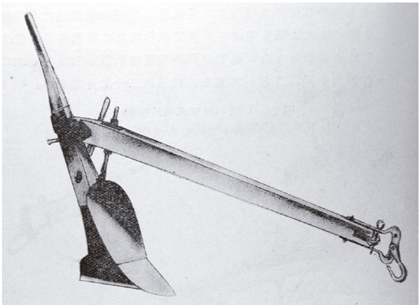
圖八、磯野犁低型號 圖片來源：臺中州立農事試驗場編，《耕鋤法》，頁22。
