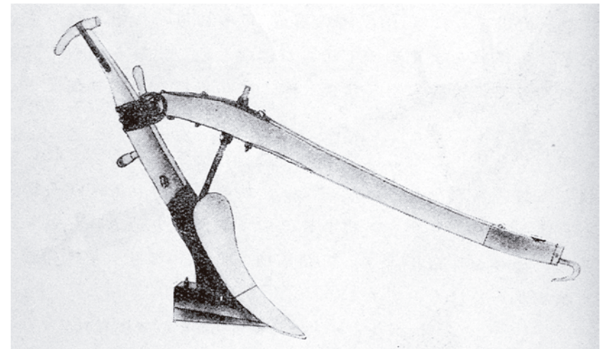
圖十五、孔明犁
